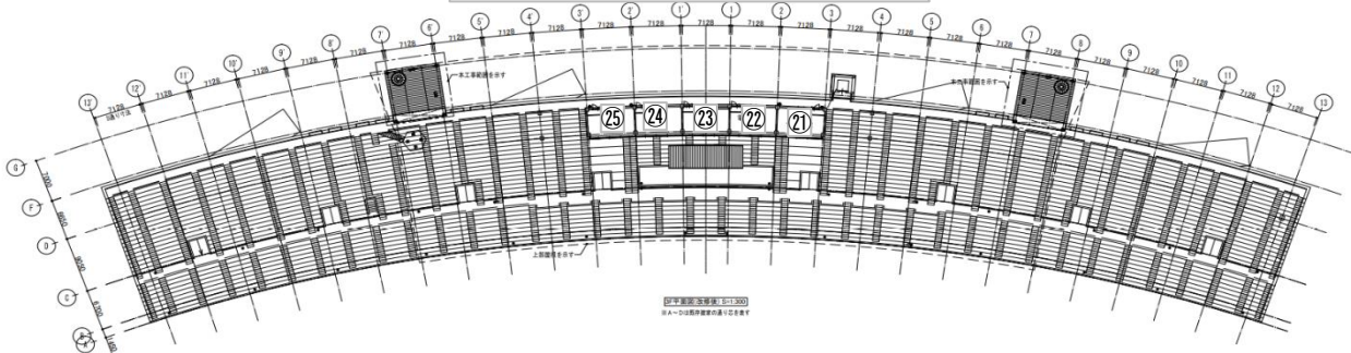
主競技場3階諸室配置図
